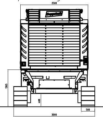
Transportstellung - Frontansicht
