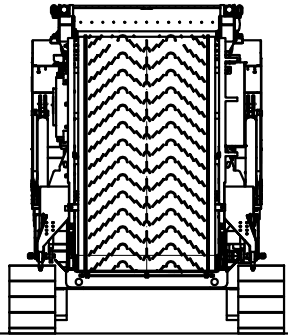
Transportstellung - Heckansicht
