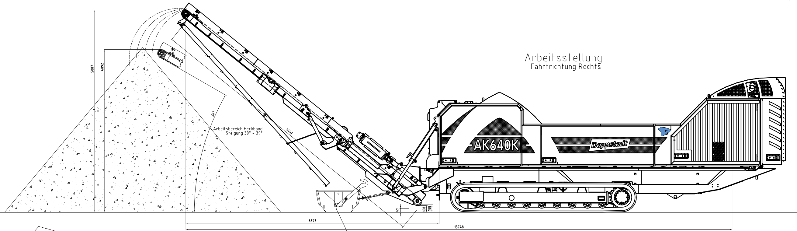
Arbeitsstellung - Draufsicht
