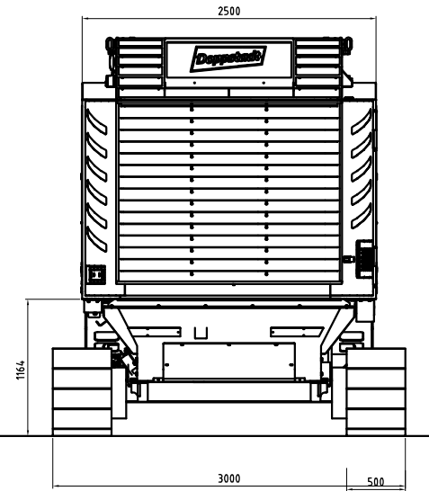
Transportstellung - Frontansicht
