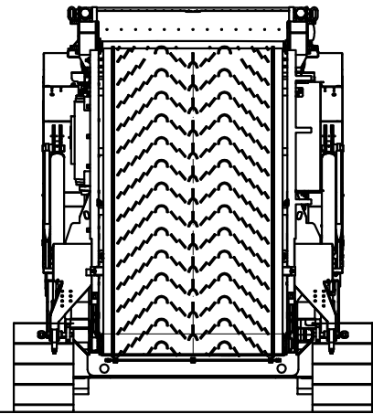
Transportstellung - Heckansicht
