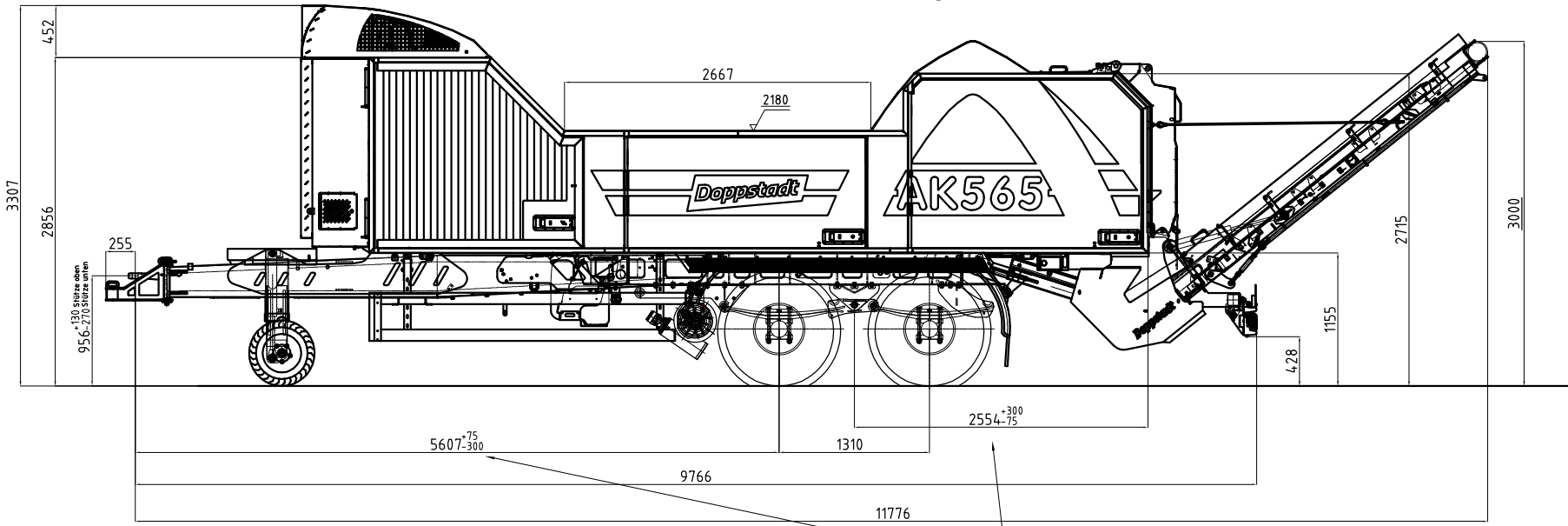
Arbeitsstellung
