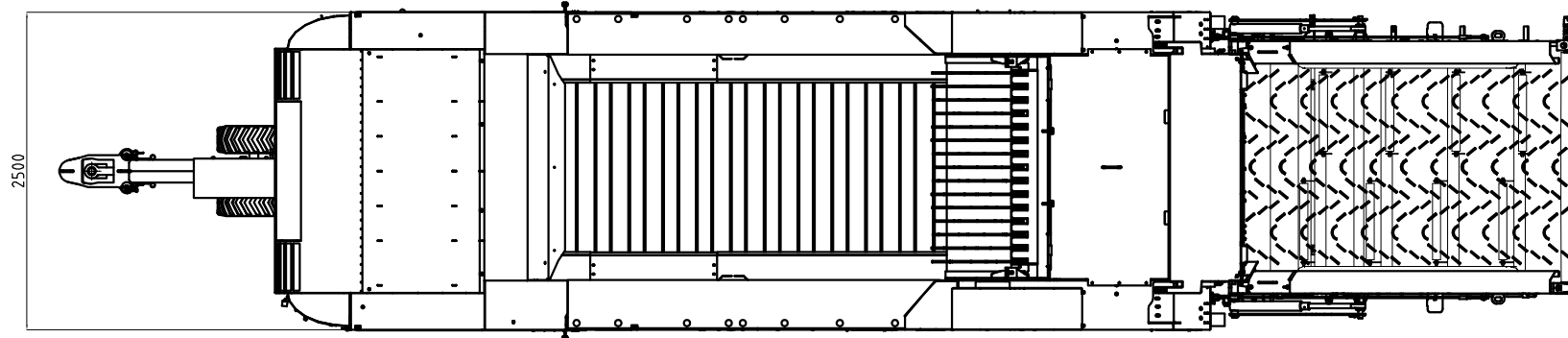
Arbeitsstellung Draufsicht
